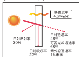
【NS70LE 施工後】
